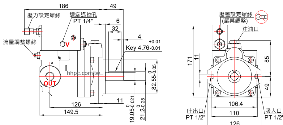
P08/10/13-BH*-F-R-TYPE
