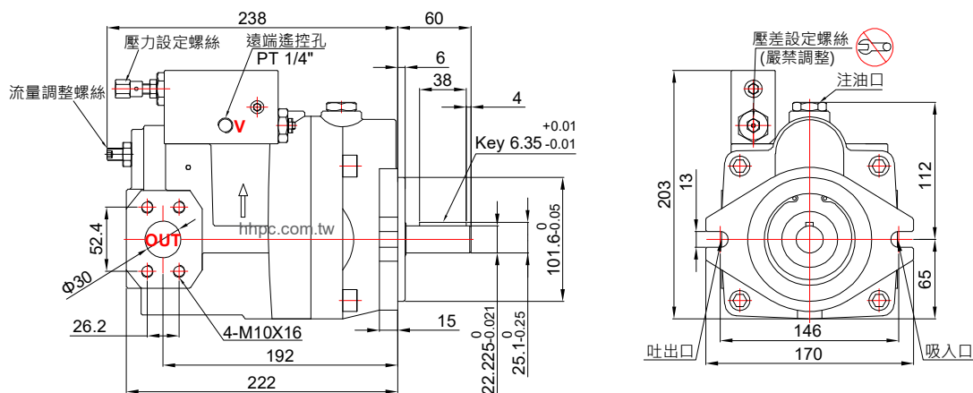
P36/46-BH*-F-R-TYPE
