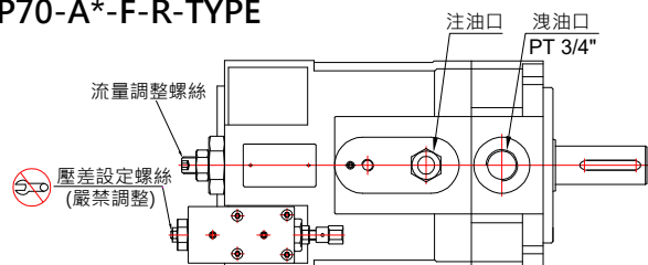
P70-A*-F-R-TYPE
